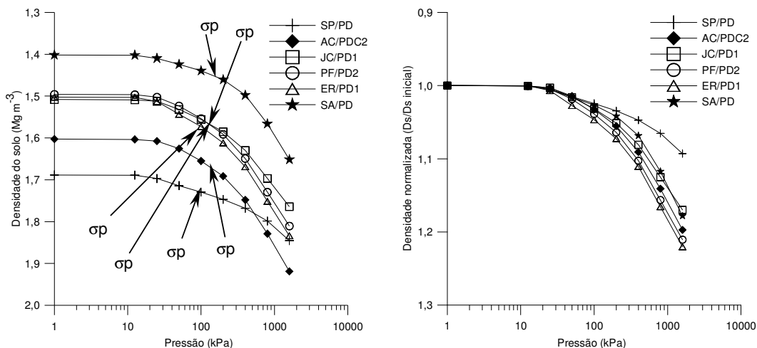
Figura 3 - Curva de compressão (esquerda) e curva de compressão normalizada (direita) para os solos em estudo.
