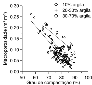
Figura 16 - Macroporosidade em função do grau de compactação para os diferentes teores de argila com densidade referência obtida pela aplicação de carga única de 1600 kPa.
