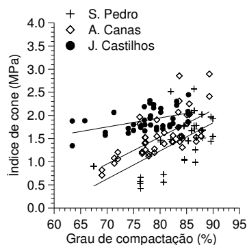
Figura 14 - Índice de cone em função do grau de compactação com densidade referência obtida com a aplicação apenas da carga de 1600 kPa para os Argissolos em estudo.
