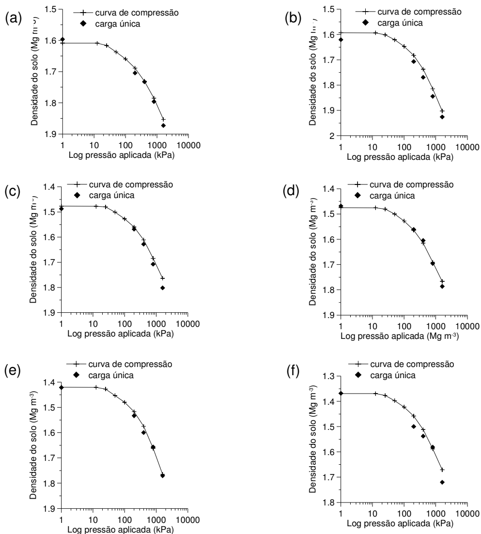
Figura 10 - Curva de compressão do solo com aplicação de cargas sucessivas e densidade do solo após aplicação de uma única carga (200, 400, 800 e 1600 kPa) em cada amostra para os solos Argissolo Vermelho distrófico arênico (u.m. São Pedro) (a), Argissolo Vermelho distrófico latossólico (u.m. Alto das Canas) (b), Argissolo Vermelho-Amarelo aluminico típico (u.m. Júlio de Castilhos) (c), Latossolo Vermelho distrófico típico (d), Latossolo Vermelho aluminoférrico típico (u.m. Erechim) (e) e Latossolo Vermelho distroférico típico (u.m. Santo Ângelo) (f).
