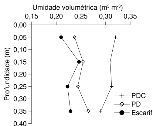
Figura 26 - Umidade volumétrica do solo ( \text{m}^3 \text{m}^{-3} ) no momento da avaliação da resistência. Avaliação realizada dia 19/09/2004 (109 dias após a semeadura do trigo).
