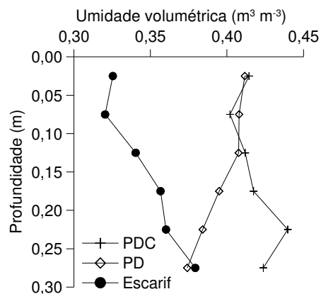
Figura 20 - Umidade volumétrica do solo ( \text{m}^3 \text{m}^{-3} ) obtida no momento da avaliação da resistência à penetração nos três tratamentos em estudo. Avaliação realizada dia 05/02/2004 (57 dias após a semeadura).
