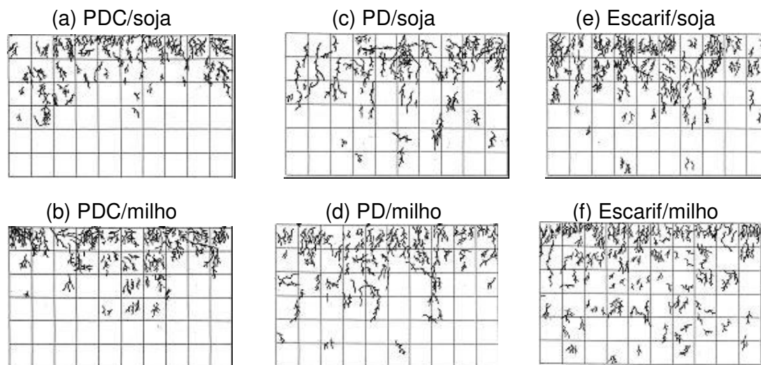
Figura 28 - Crescimento radicular da cultura do trigo nos diferentes níveis de compactação (PDC, PD e Escarif) e sucessão de culturas (soja/milho). Malha de 0,05 m x 0,05 m. Avaliação realizada dia 19/09/2004 (109 dias após a semeadura do trigo).
