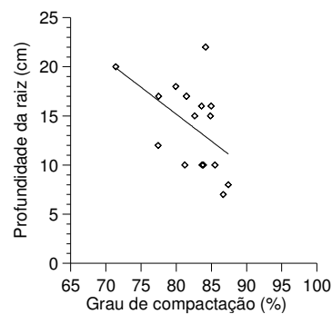
Figura 17 - Profundidade de raiz em função do grau de compactação para os diferentes teores de argila com densidade referência obtida com a aplicação de carga única de 1600 kPa.
