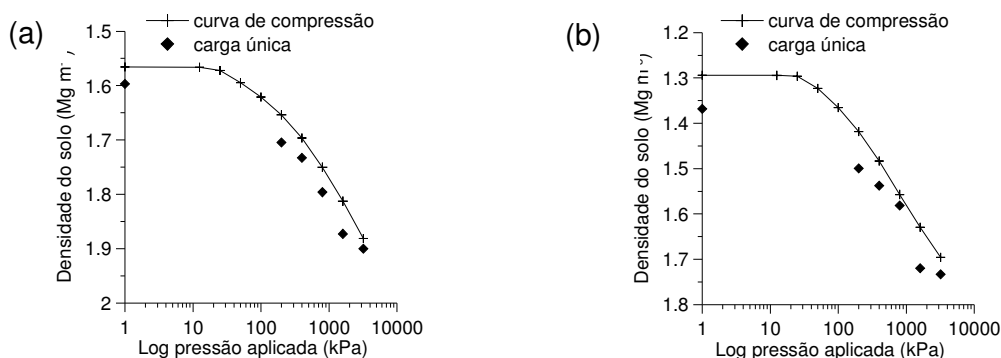
Figura 11 - Curva de compressão do solo com aplicação de cargas sucessivas e densidade do solo após aplicação de uma única carga (200, 400, 800, 1600 e 3200 kPa) em cada amostra para os solos Argissolo Vermelho distrófico arênico (u.m. São Pedro) (a) e Latossolo Vermelho distroférico típico (u.m. Santo Ângelo) (b).
