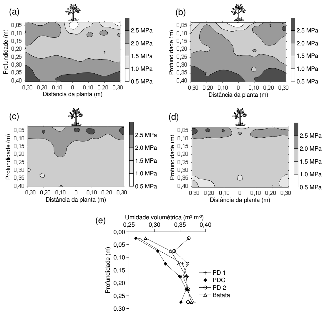
Figura 6 - Resistência à penetração do Argissolo Vermelho-Amarelo aluminico típico nos manejos PD 1 (a), PDC (b), PD 2 (c) e Batata (d), e umidade do solo (e) no momento da avaliação da resistência.
