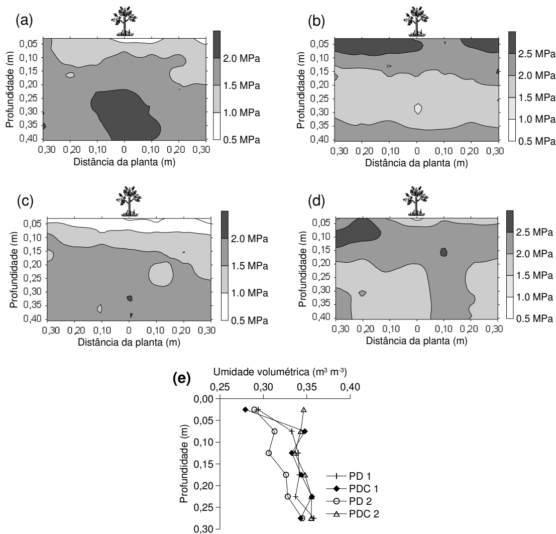
Figura 7 - Resistência à penetração do Latossolo Vermelho distrófico típico nos manejos PD 1 (a), PDC 1 (b), PD 2 (c) e PDC 2 (d), e umidade do solo (e) no momento da avaliação da resistência.
