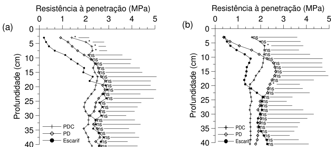
Figura 19 - Resistência à penetração do solo na cultura da soja (a) e milho (b) nos três tratamentos em estudo. Avaliação realizada dia 05/02/2004 (57 dias após a semeadura). Barras horizontais comparam os valores de resistência à penetração para cada profundidade, pelo teste DMS a 5%.
