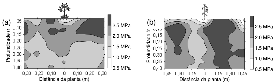
Figura 21 - Resistência à penetração no tratamento PDC, nas culturas da soja (a) e milho (b). Avaliação realizada dia 19/04/2004 (131 dias após a semeadura).
