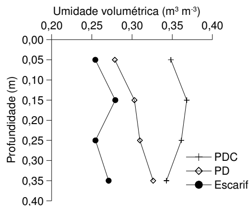
Figura 24 - Umidade volumétrica do solo ( \text{m}^3 \text{m}^{-3} ) no momento da avaliação da resistência do solo à penetração nos tratamentos em estudo. Avaliação realizada dia 19/04/2004 (131 dias após a semeadura).
