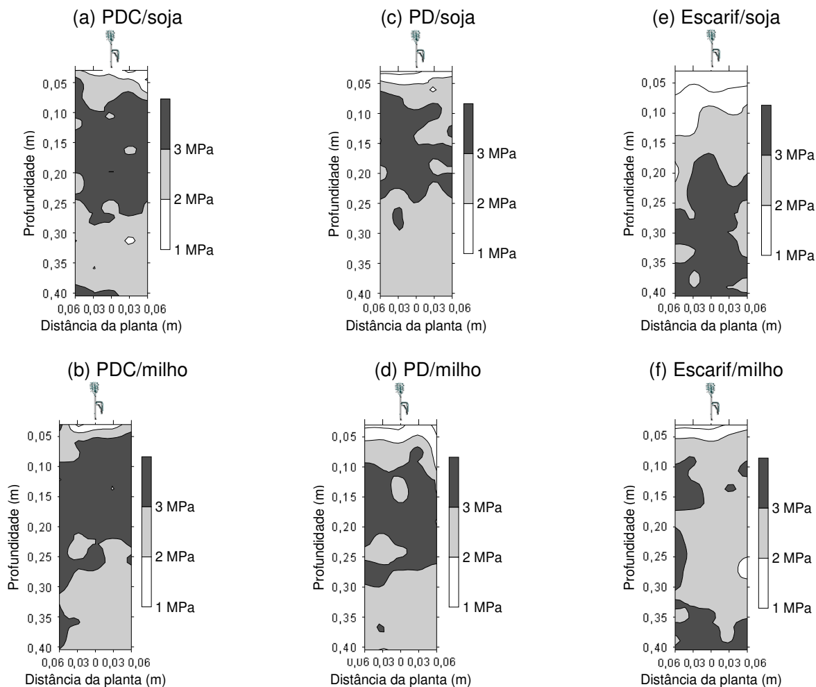
Figura 27 - Resistência do solo à penetração nos diferentes níveis de compactação (PDC, PD e Escarif) e sucessão de culturas (soja/milho). Avaliação realizada dia 19/09/2004 (109 dias após a semeadura do trigo).
