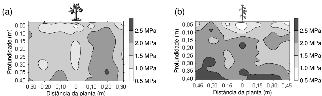
Figura 22 - Resistência à penetração no tratamento PD, nas culturas da soja (a) e milho (b). Avaliação realizada dia 19/04/2004 (131 dias após a semeadura).
