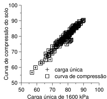
Figura 12 - Grau de compactação utilizando densidade referência obtida com a carga de 1600 kPa da curva de compressão em função do grau de compactação obtido com a densidade referência aplicando apenas 1600 kPa.
