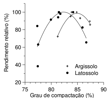
Figura 13 - Rendimento relativo em função do grau de compactação com densidade referência obtida com aplicação apenas da carga de 1600 kPa para os Argissolos e Latossolos em estudo.
