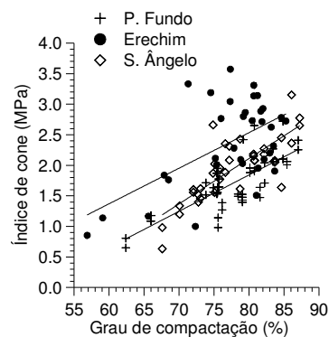
Figura 15 - Índice de cone em função do grau de compactação com densidade referência obtida com a aplicação apenas da carga de 1600 kPa para os Latossolos em estudo.
