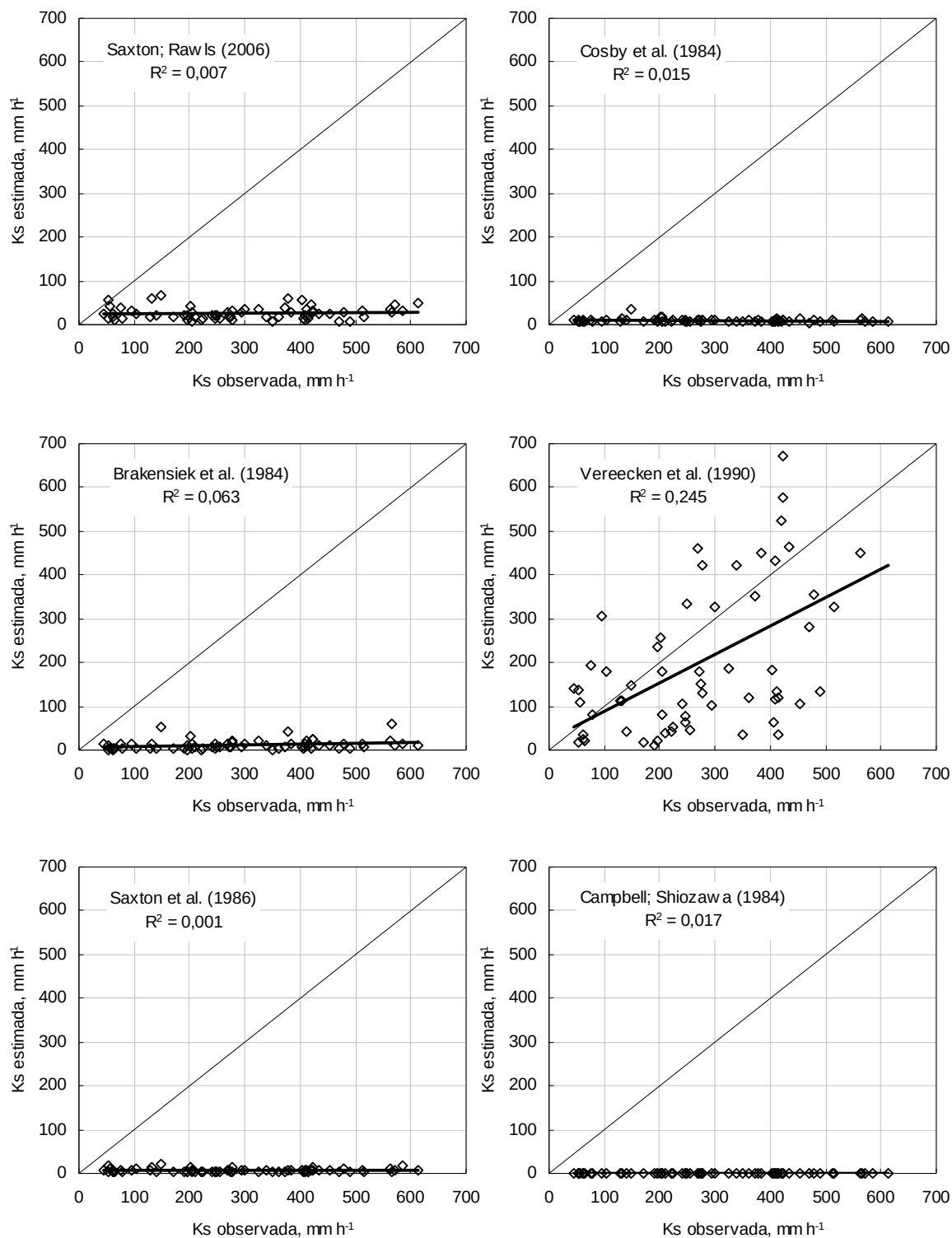
Figura 12 – Relação 1:1 dos valores de condutividade hidráulica do solo saturado ( K_s ) observados nos pontos amostrados da microbacia e os estimados pelas funções de pedotransferência encontradas na literatura.
