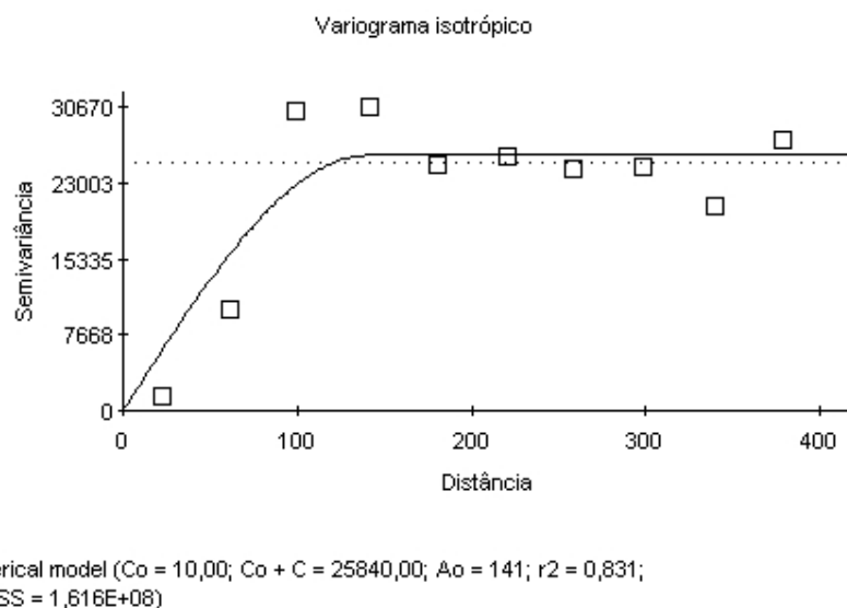
Figura 8 – Modelo de semivariograma (esférico) ajustado para os dados coletados no solo da microbacia. Co = efeito pepita; Co + C = patamar; Ao = alcance; r2 ( R^2 ) = coeficiente de determinação; RSS = soma de quadrados de resíduos.
