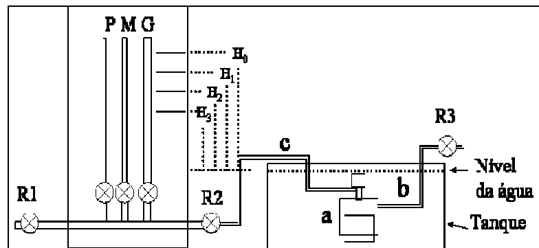
Figura 4 – Esquema do permeâmetro utilizado na determinação da condutividade hidráulica de solo saturado. Fonte: Gubiani et al., 2008.
