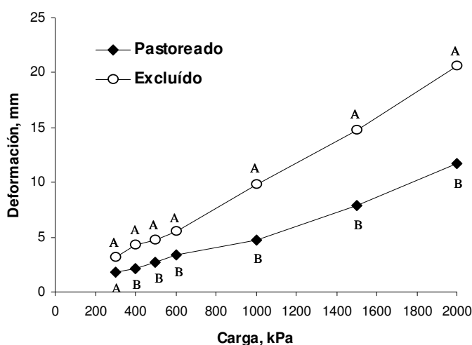
Figura 8 - Deformación del suelo con contenido de agua volumétrico en el suelo de 39 %, frente a diferentes presiones en suelo excluido de pastoreo y pastoreado, en el ensayo 1. Letras diferentes indican diferencias significativas según ANOVA.
