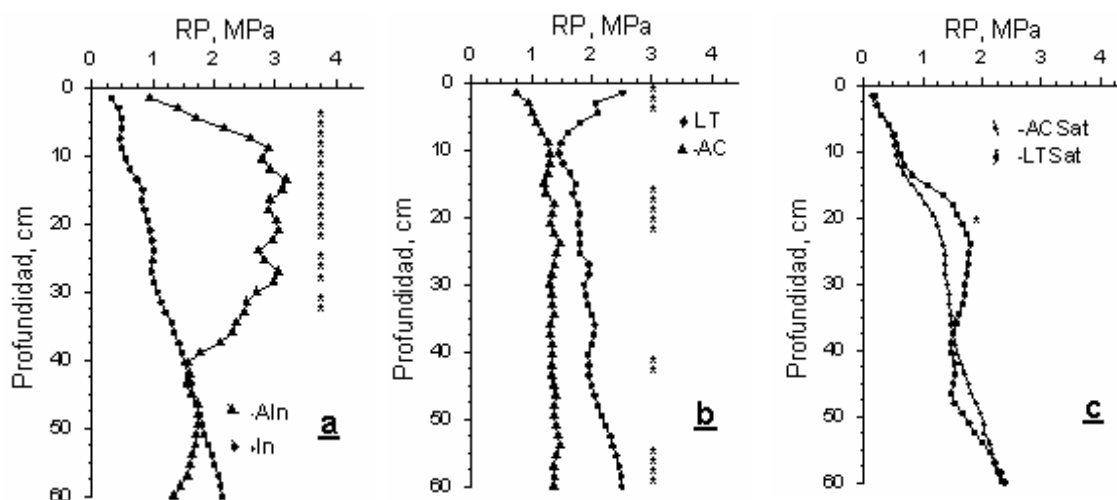
Figura 13 - Resistencia a la penetración en suelo bajo cultivo de arroz, a – antes de inundar el área (AIn) el 5/12/1999 con 22% de humedad y después de inundado (In) el 15/01/2000, suelo saturado; b – antes de la cosecha de arroz (AC), el 15/3/2000, suelo con 25% de humedad, y en la huella (LT) de la cosechadora, suelo con 25% de humedad ; c – antes de la cosecha de arroz, el 25/3/2001, suelo saturado (ACSat) y en la huella de la cosechadora (LTSat), suelo saturado. (*Significativo al 5 %).
