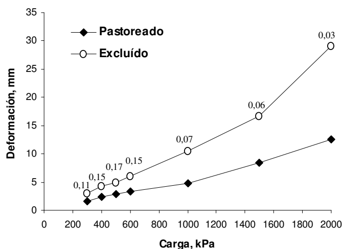
Figura 9 - Deformación del suelo con contenido de agua volumétrico en el suelo de 39 %, frente a diferentes presiones, en suelo excluido de pastoreo y pastoreado, en el ensayo 2. Se presentan los valores de Prueba T, Prob de error Tipo 1.
