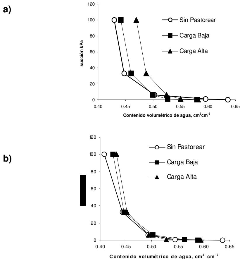
Figura 6 - Curva característica de agua en el suelo en las profundidades de 0 - 3 cm (a) y 9 – 12 cm (b), en el experimento 2.
