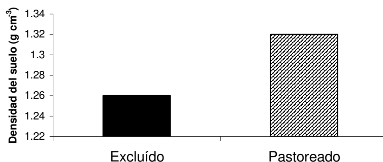
Figura 5 - Valores de densidad del suelo por el método del terrón parafinado, en suelo excluido y pastoreado (compactado) en experimento 1, en la profundidad de 0 8 cm.
