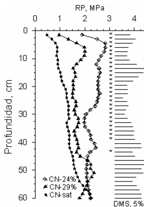
Figura 15 - Resistencia a la penetración en suelo bajo campo natural a diferentes condiciones de humedad del suelo.
