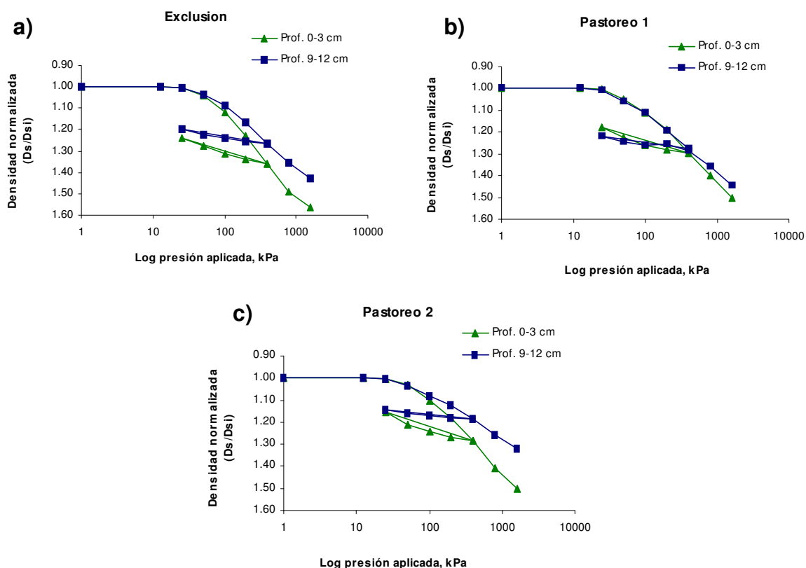
Figura 10 - Curva de compresión y recompresión del suelo para los tratamientos en estudio, Exclusión (a), Pastoreo 1 (b), Pastoreo 2 (c) en las profundidades de 0-3 y 9-12 cm. D_{si} = D_s inicial.
