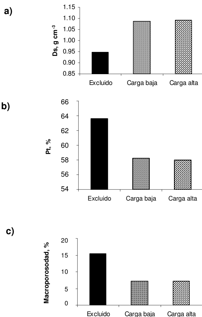
Figura 7 - Valores de densidad del suelo D_s (a), porosidad total P_t (b) y macroporosidad (c), en el ensayo 2, en la profundidad de 0 – 3 cm.
