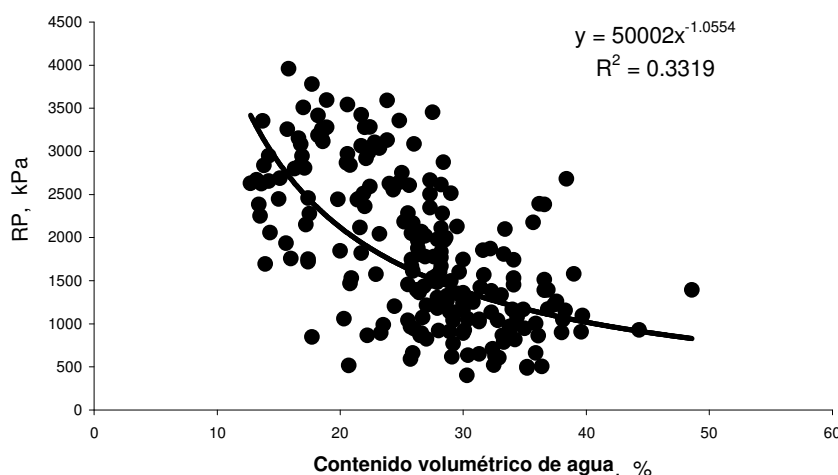
Figura 11 - Relación entre la resistencia a la penetración (RP) y el contenido de agua volumétrico en el suelo hasta 6 cm de profundidad.
