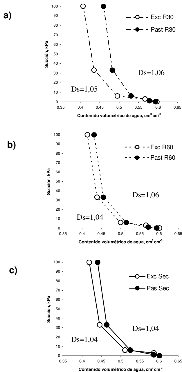
Figura 4 - Curvas características de retención de agua y densidad del suelo ( D_s ), de los tratamientos de Riego R30 (a), R 60 (b) y secano (c), bajo exclusión de pastoreo (Exc) y con pastoreo (Past) en el experimento 1 en la profundidad de 0 – 3 cm.
