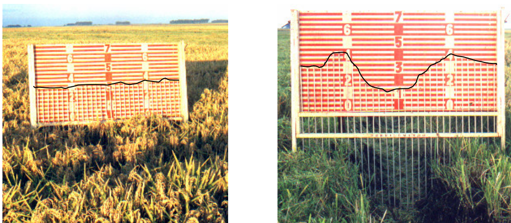
Figura 14 - Imágenes de perfilómetro en condición de cultivo de arroz, antes de la cosecha (izquierda) y post cosecha, en la huella de la rueda de la cosechadora (derecha).
