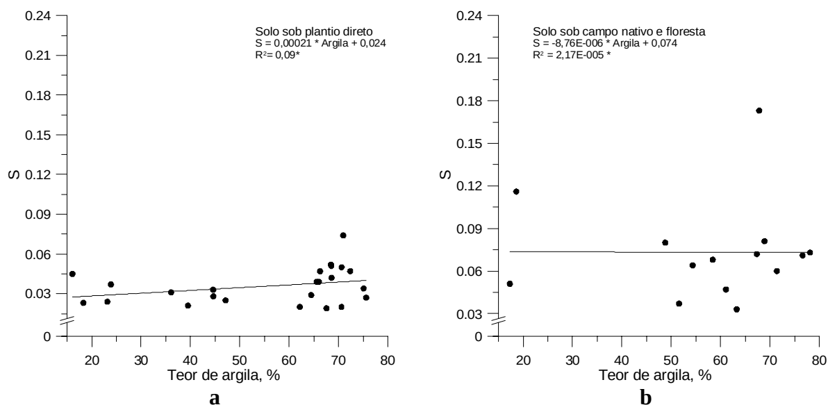
Figura 3 – Comportamento do índice S em função do teor de argila para solos sob diferentes usos (* o modelo ajustado não é significativo a p \leq 0,01 pelo teste F)
