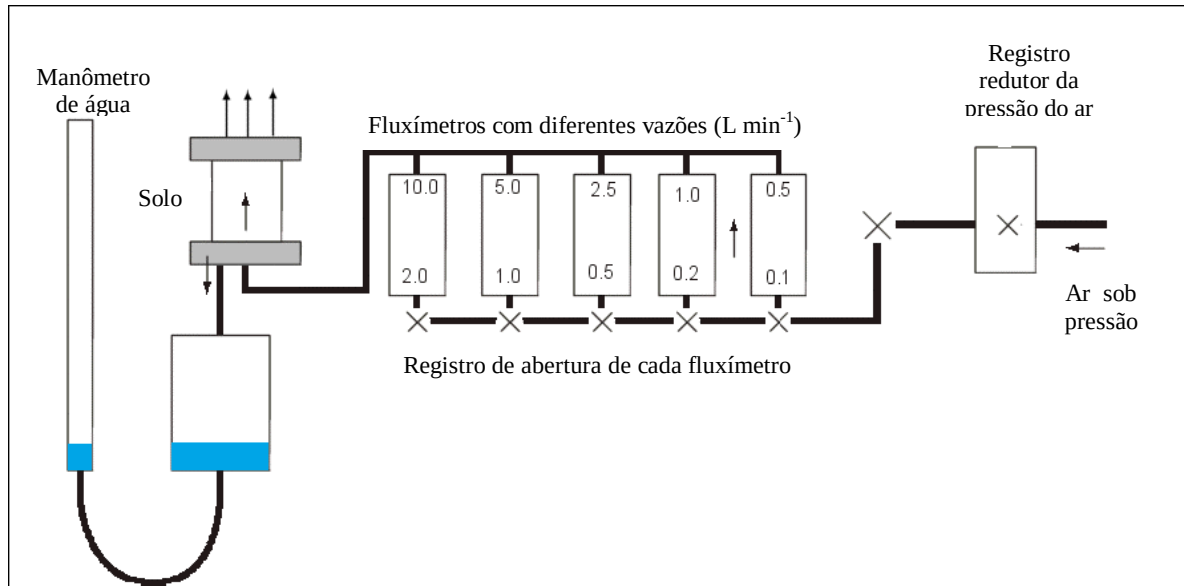
Figura 9 – Permeâmetro utilizado para determinação da condutividade do ar no solo ( K_l ) em amostras de estrutura preservada
